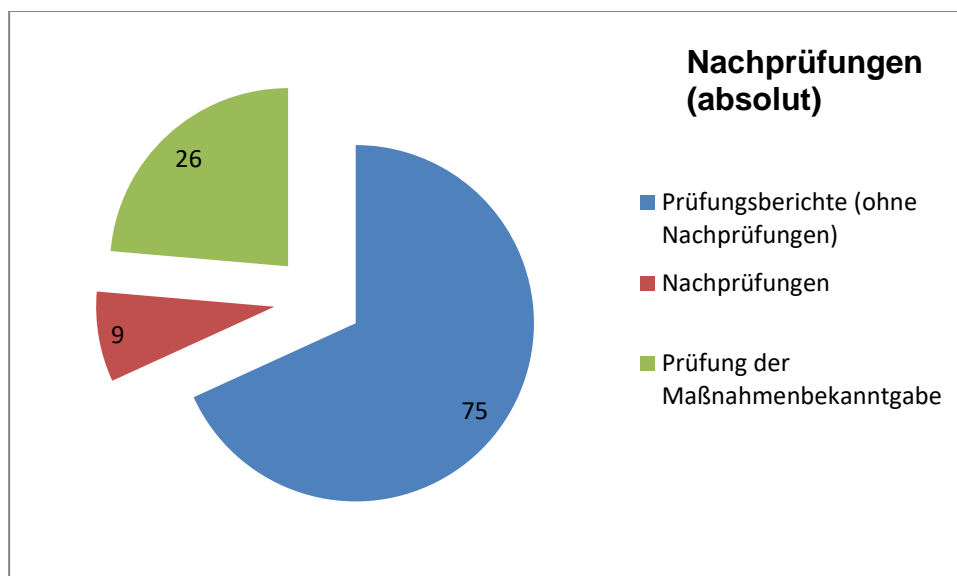
Abbildung 3: Nachprüfungen (absolut)
